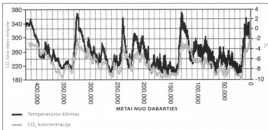
KLIMATO SVYRAVIMAI PER PASTARUOSIUS 420 000 M., PAGAL „VOSTOK“ STOTIES ANTARKTIDOJE KERŲ
