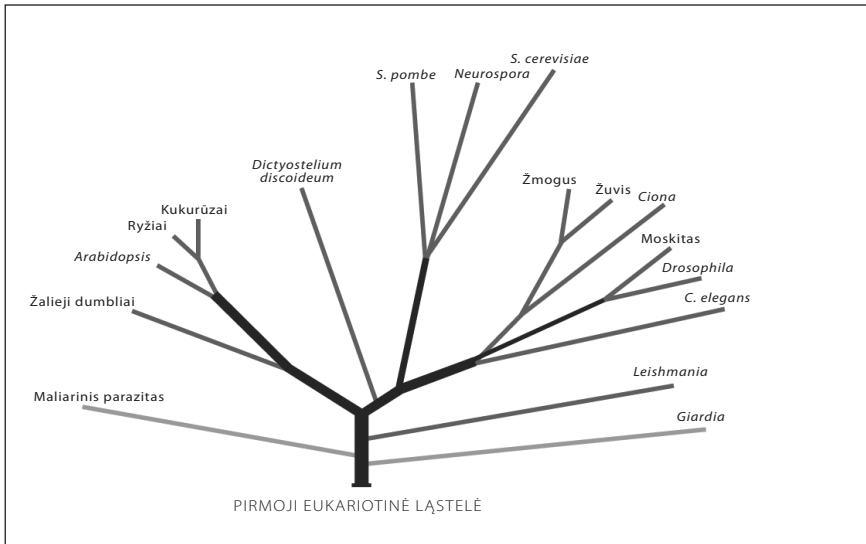
4.2 PAV. ĮPRASTAS GYVYBĖS MEDIS, RODANTIS EUKARIOTINIŲ ORGANIZMŲ DIVERGENCIJĄ NUO BENDROJO PROTĖVIO – VIENALĄSČIO ORGANIZMO, GYVENUSIO MAŽDAUG PRIEŠ 2 MLRD. M. KUO ILGESNĖ ŠAKA, TUO DIDESNIS EVOLIUCINIS ATSTUMAS, T. Y. TUO SKIRTINGESNI GENAI.
