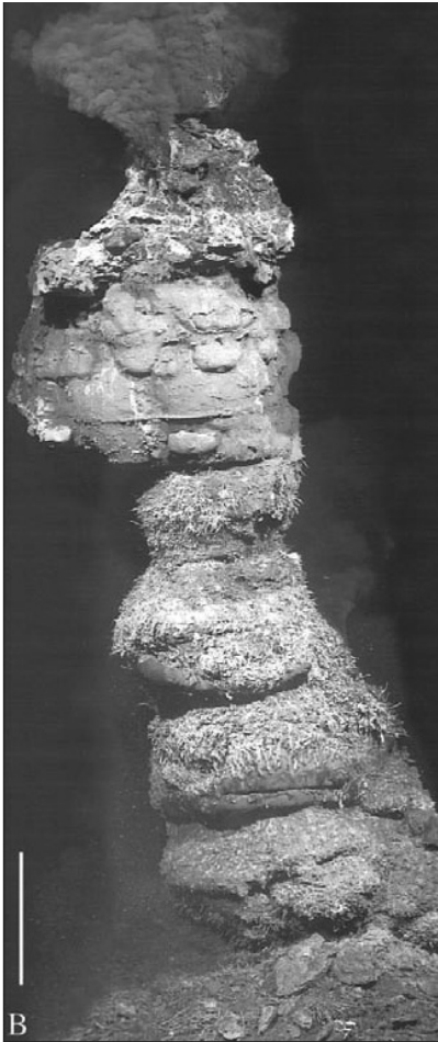
1.1 PAV. VULKANINIS JUODASIS RŪKALIUS, LEIDŽIANTIS 350 °C TEMPERATŪROS VANDENĮ TIES CHUAN DE FUKOS TEKTONINĖS PLOKŠTĖS KRAŠTU RAMIOJO VANDENYNŲ ŠIAURĖS RYTUOSE. ŽYMEKLIS YRA 1 M AUKŠČIO.
