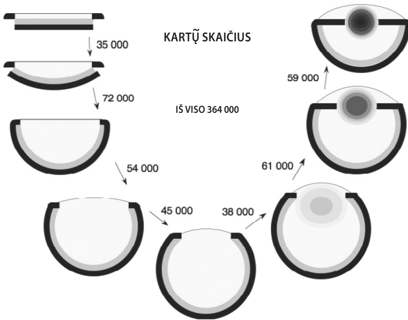
7.2 PAV. D. E. NILSONO IR S. PELGER SUDARYTA SEKA ETAPŲ, KURIŲ REIKIA, KAD IŠSIVYSTYTŲ AKIS, IR ATITINKAMAS KARTŲ SKAIČIUS, PER KURĮ ĮSITVIRTINA KIEKVIENAS POKYTIS. DARANT PRIELAIĐĄ, KAD KIEKVIENA KARTA PRILYGSTA 1 M., VISAS TOKS VYSTYMASIS UŽTRUNKA KIEK MAŽIAU NEI 0,5 MLN.M.
